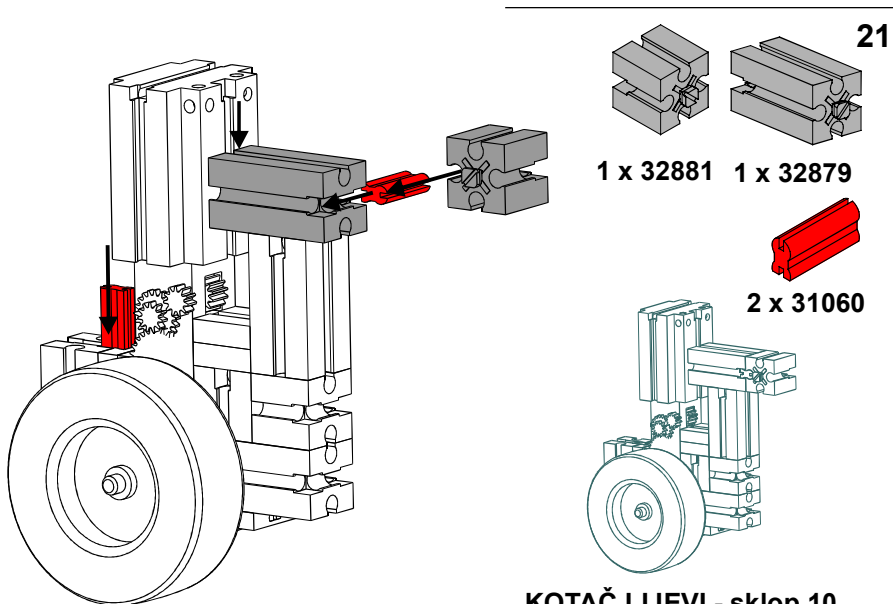
KOTAČ LIJEVI - sklop 10
